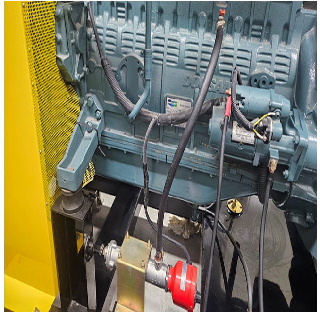
히터호스 교체 완료
